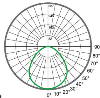
Cd Curva correspondiente de 90°, 270° horizontales
