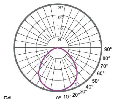
Cd Curva correspondiente de 45°, 225° horizontales
